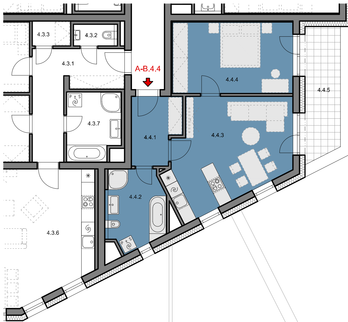
PŮDORYS 1:100
