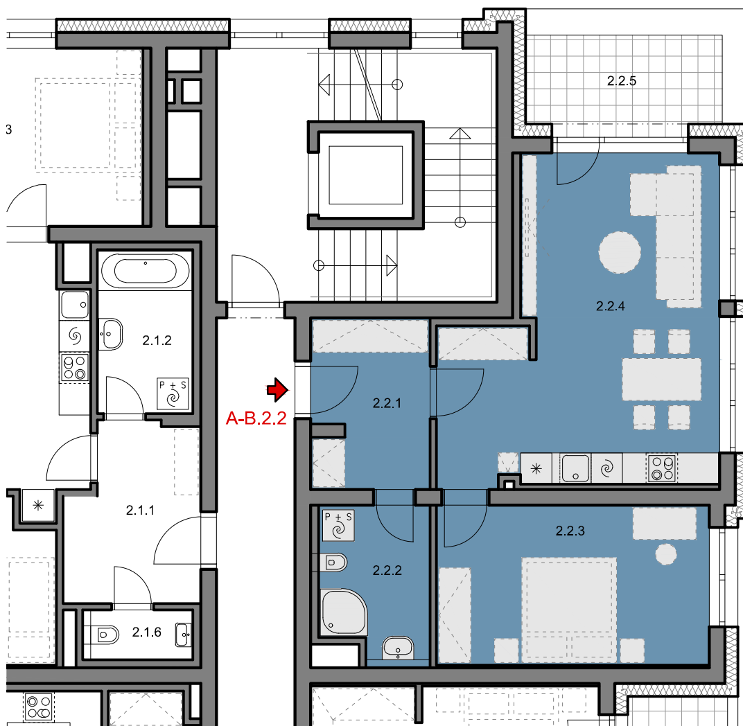
PŮDORYS 1:100
