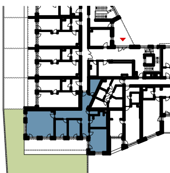
SCHÉMATICKÝ PŮDORYS
