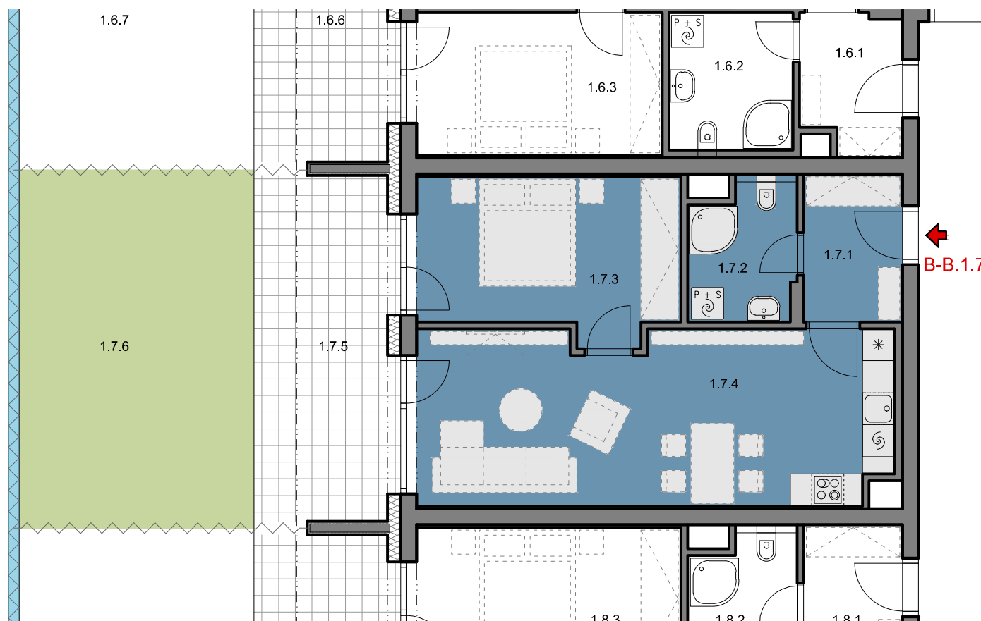
PŮDORYS 1:100
